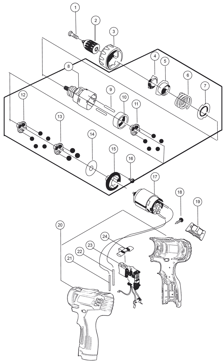
Схема и детали сборки ДША-12ЛБ
