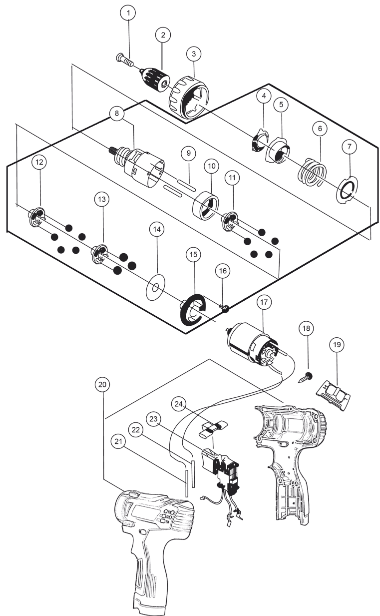
Схема и детали сборки VDS-10/12L
