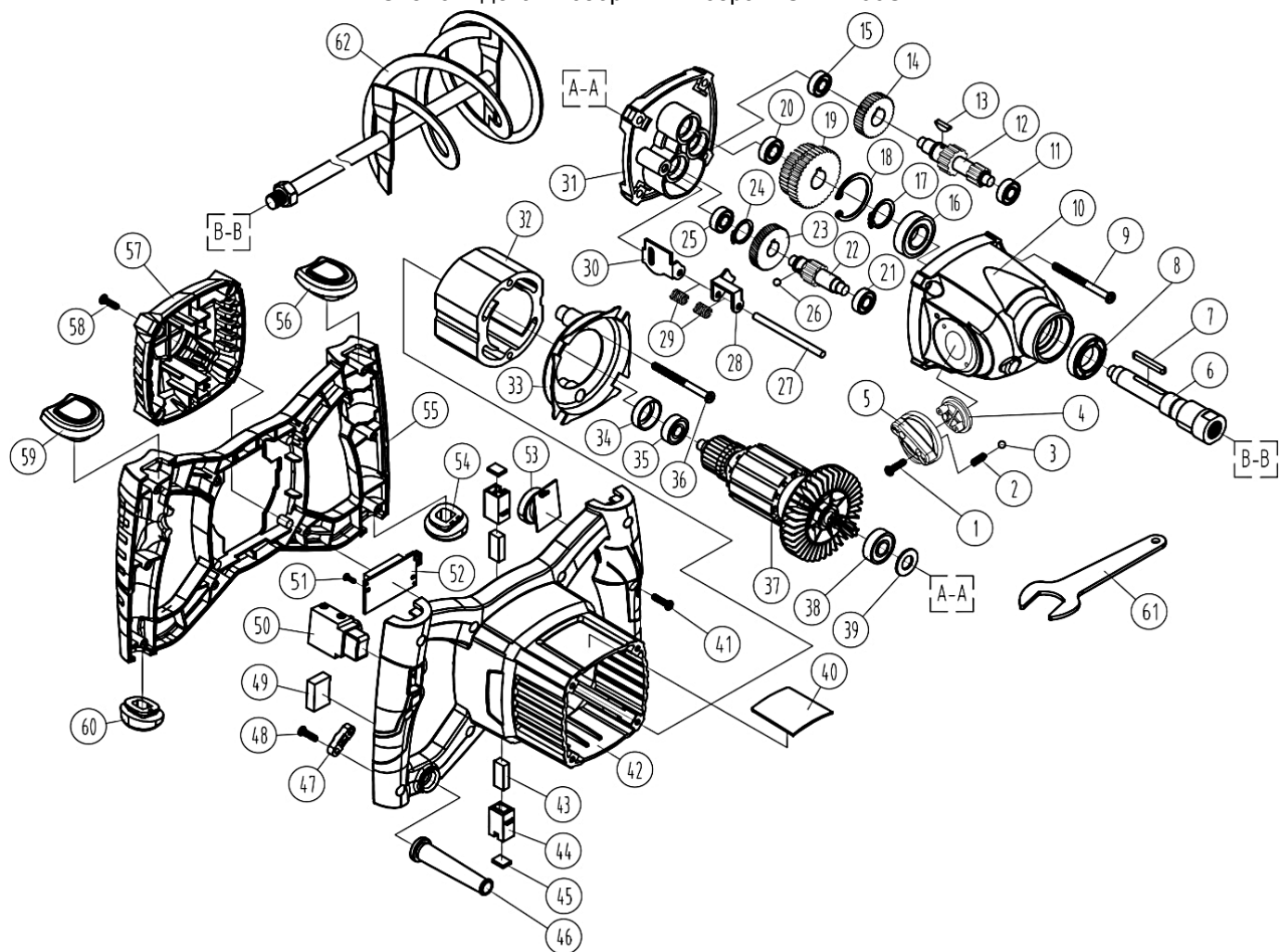
Схема и детали сборки миксера МЭ-2 1400ЭМ
