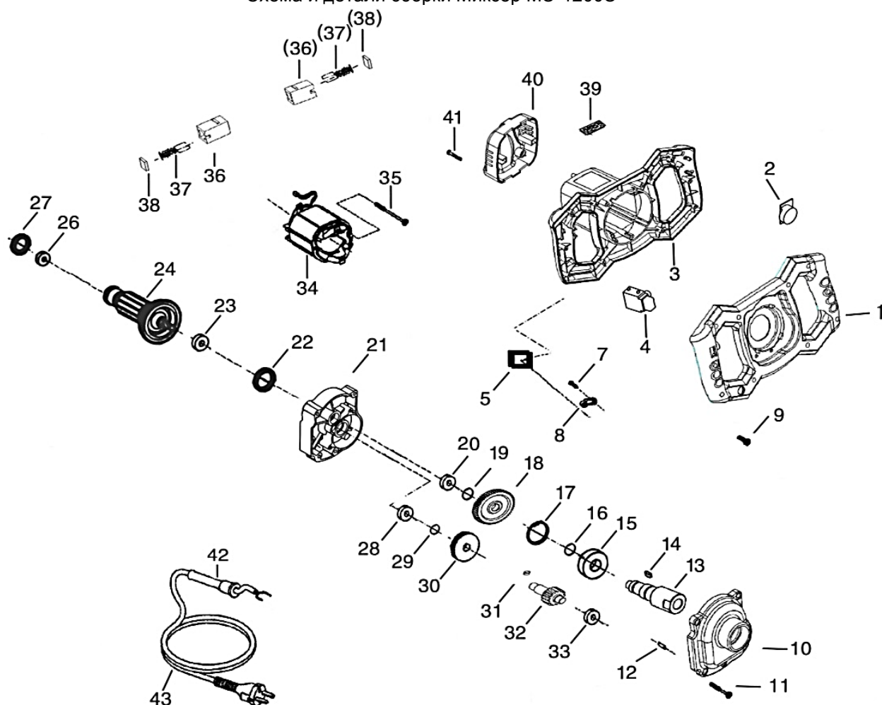
Схема и детали сборки Миксер МЭ-1200Э
