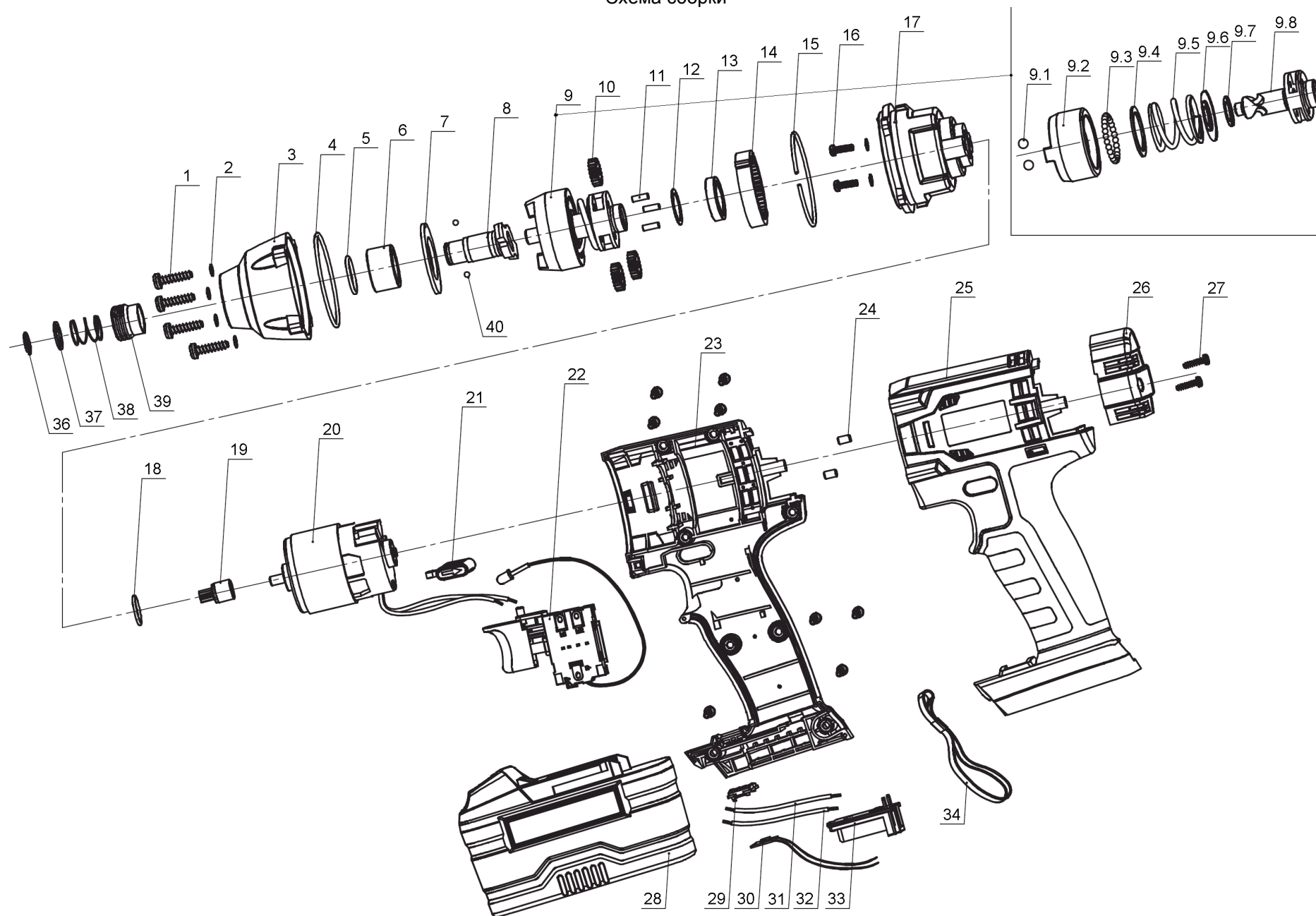
Схема сборки
