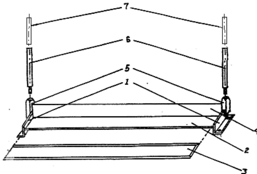
Схема сборки «КОРВЕТ 501»
