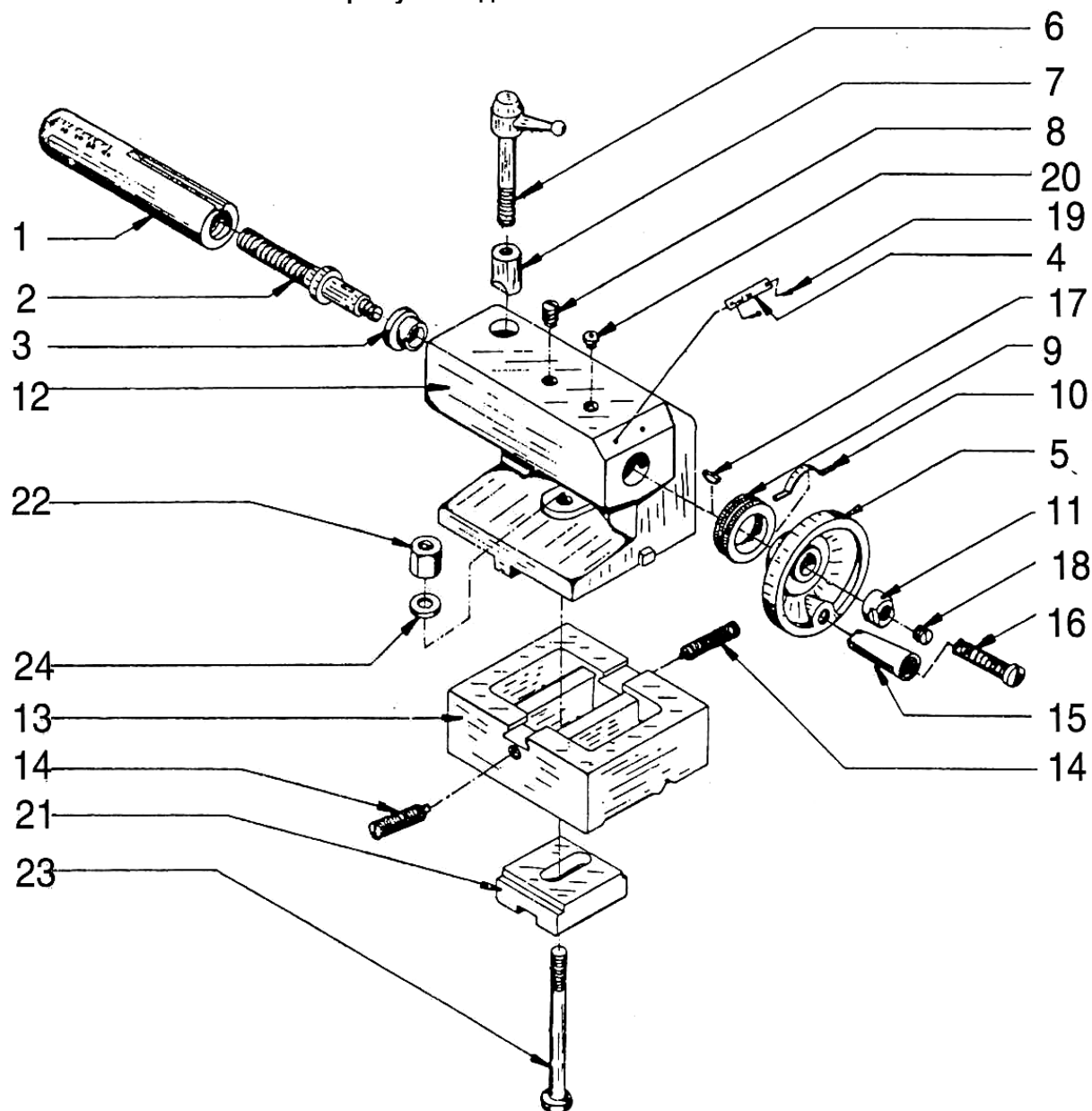
Схема сборки узла задней бабки станка «КОРВЕТ 402»
