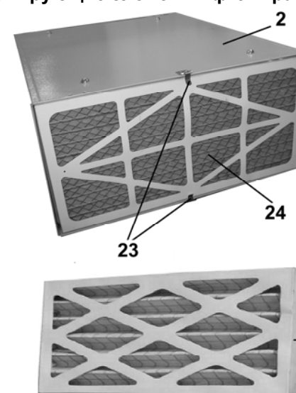
2 - Корпус 23 - Фиксатор
