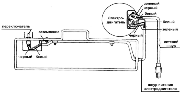
Электрическая схема
